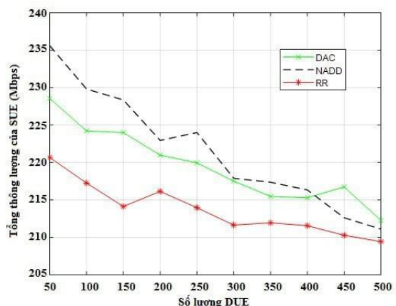
Hình 3. Thông lượng của kết nối SUE
