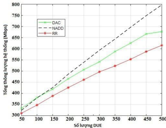
Hình 5: Thông lượng hệ thống
