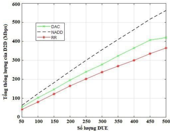
Hình 4. Thông lượng của các kết nối D2D
