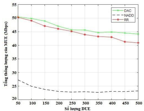
Hình 2. Thông lượng của các kết nối MUE
