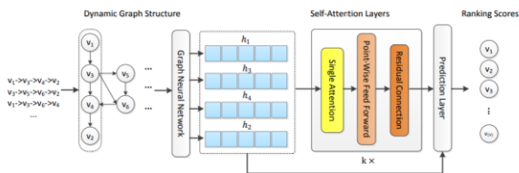
Hình 3. Kiến trúc GC-SAN
