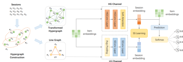
Hình 4. Kiến trúc DHCN
