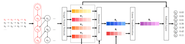
Hình 1. Kiến trúc SR-GNN
