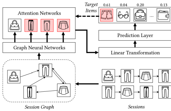
Hình 2. Kiến trúc TA-GNN
